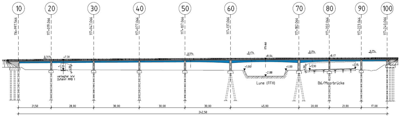
Ansicht des Bauwerkes im Zuge der A 27 über die Lune und die B 6 im Abschnitt 4
